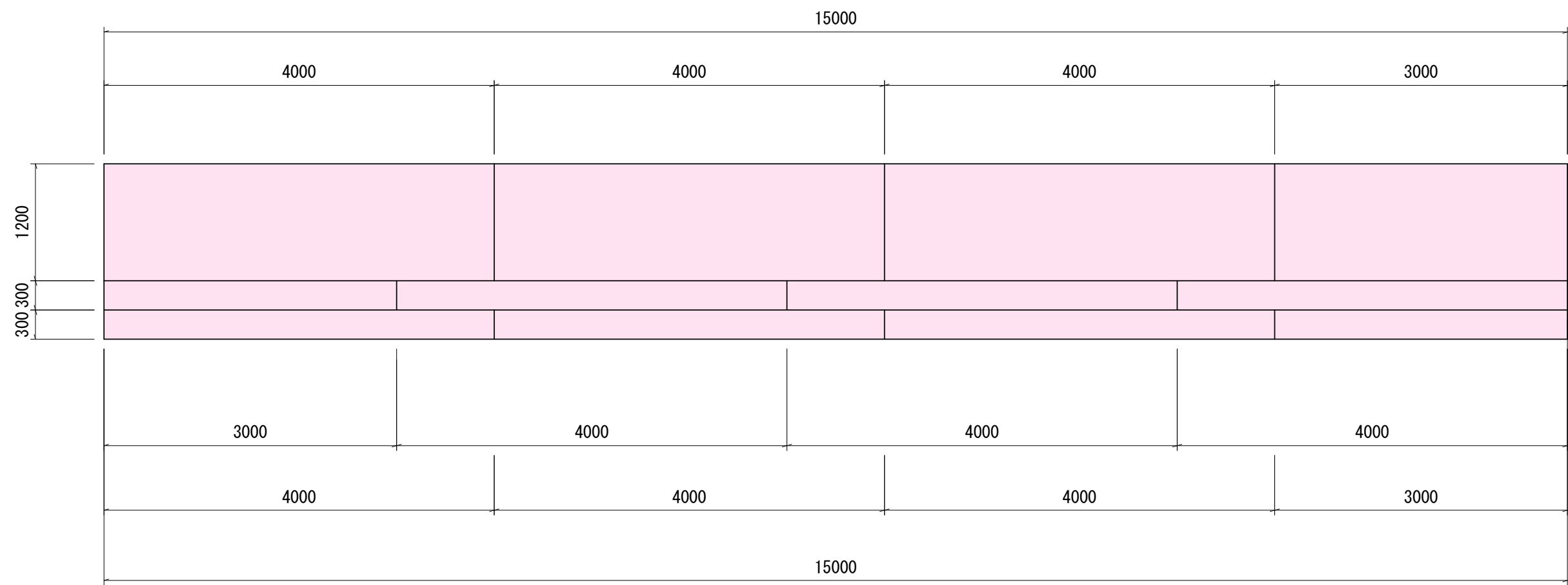
正 面 図
