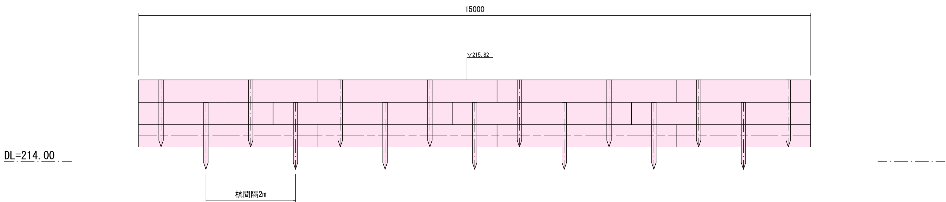
正 面 図
