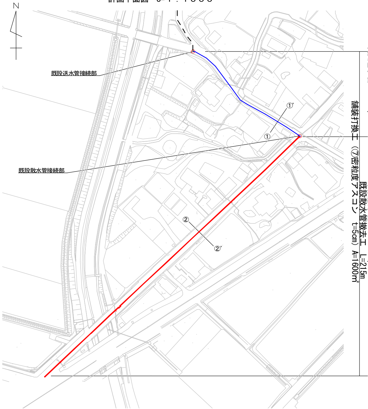
計画平面図 S=1:1000
