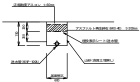
送水管布設部標準断面
