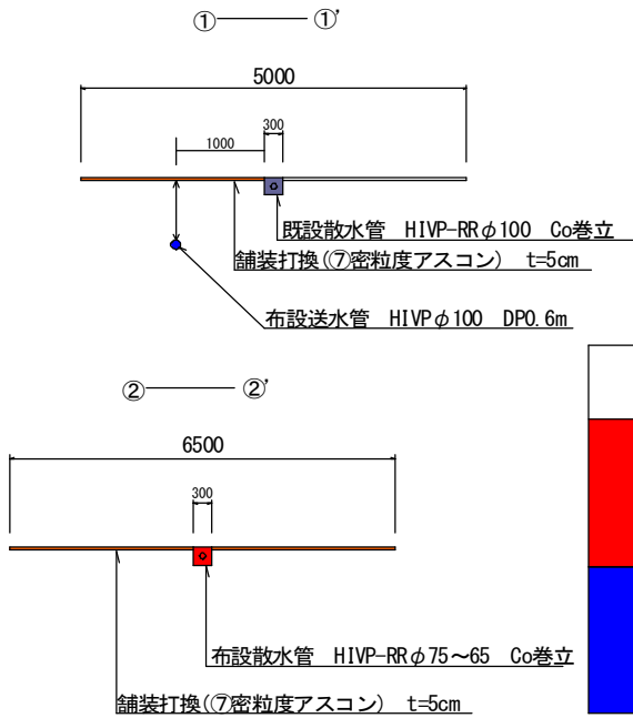
標準横断面図 S=Free
