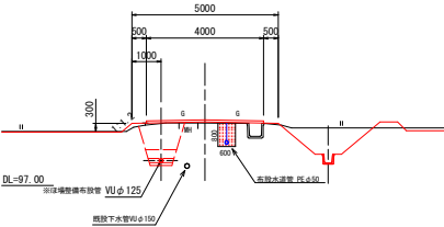
標準断面図 S=1:100
