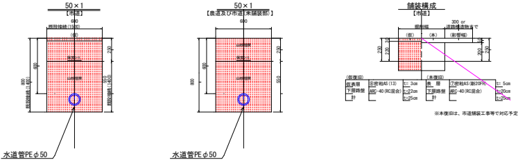
掘削標準断面図 1:20
