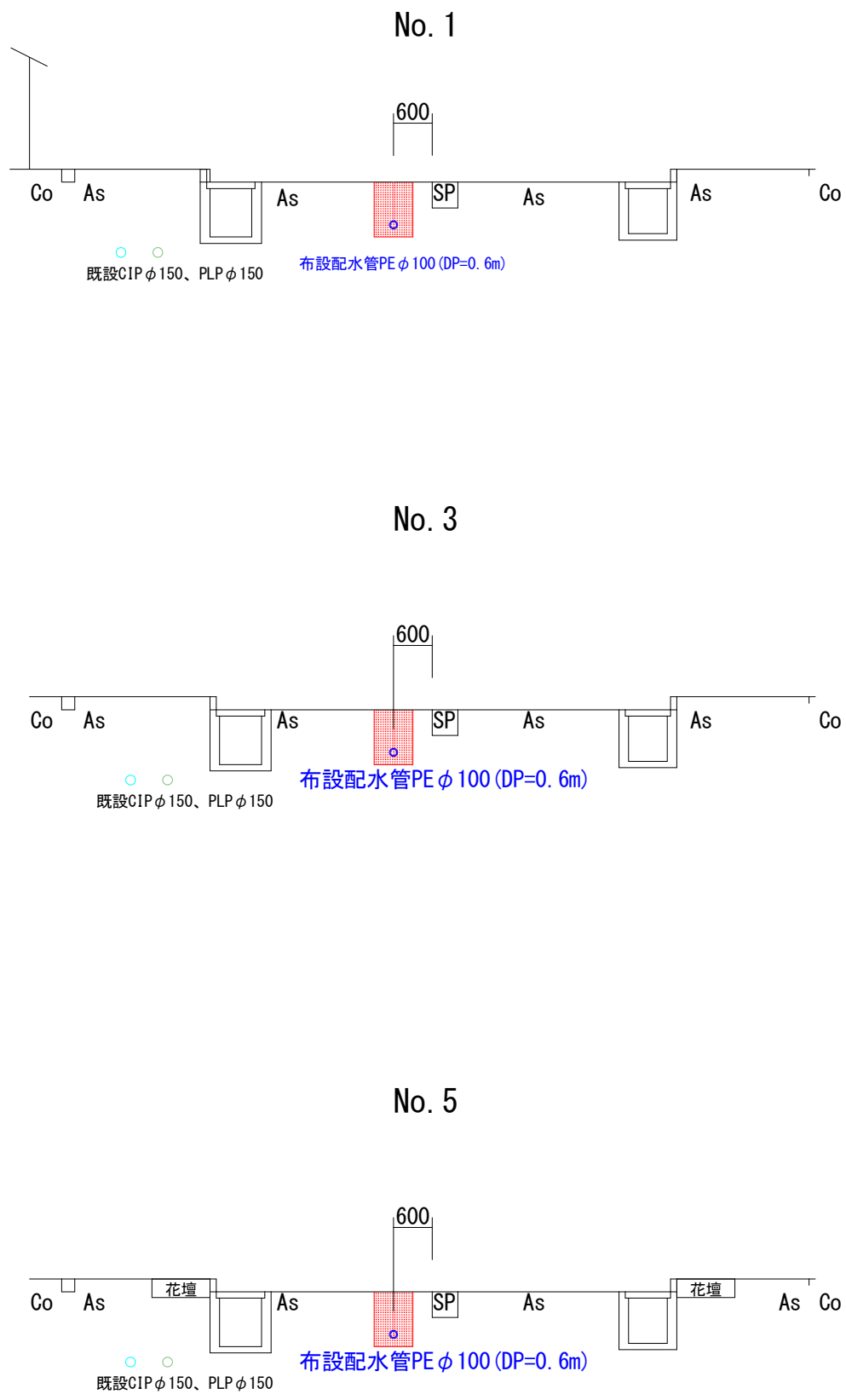
標準横断面図 1:100
