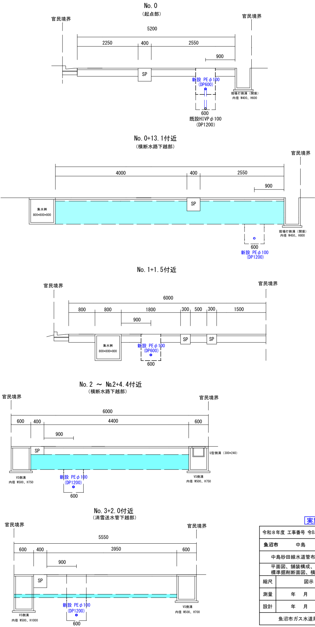
横断面図 S=1:50
