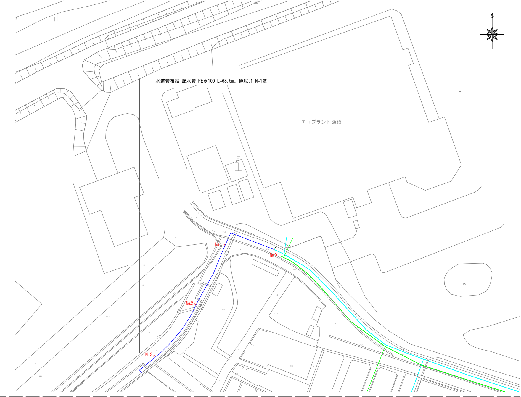
平面図 1:500
