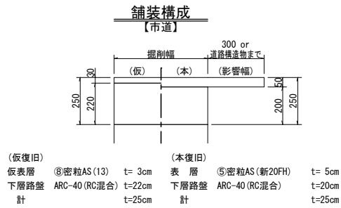
舗装構成 S=1:20
