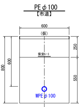
標準掘削断面図 S=1:20
