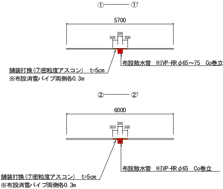
標準横断面図 S=Free
