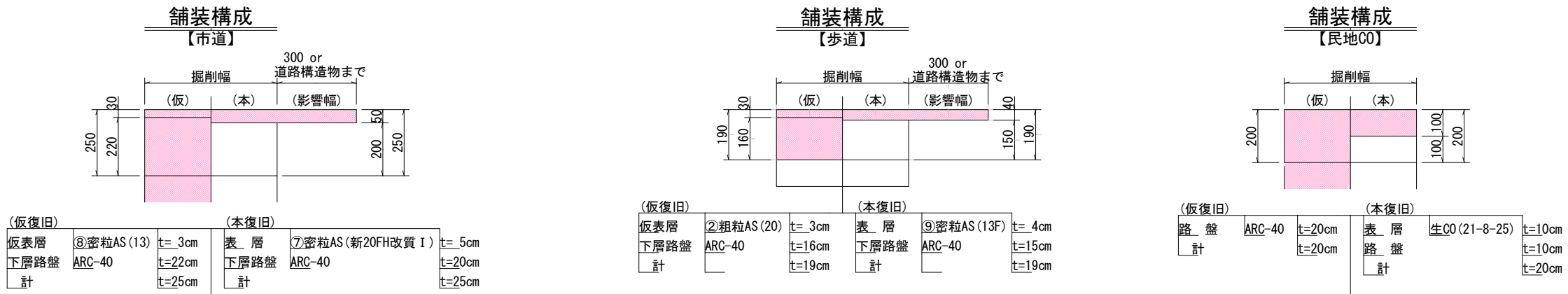
舗装構成図 S=1:20
