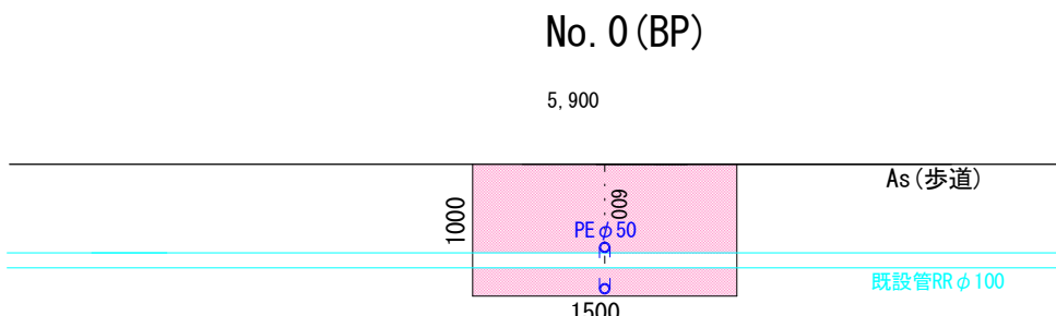
横断面図 S=1:50
