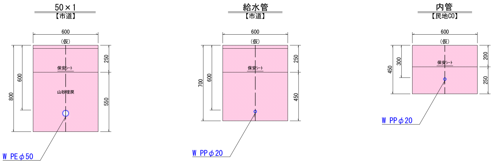
掘削標準断面図 S=1:20
