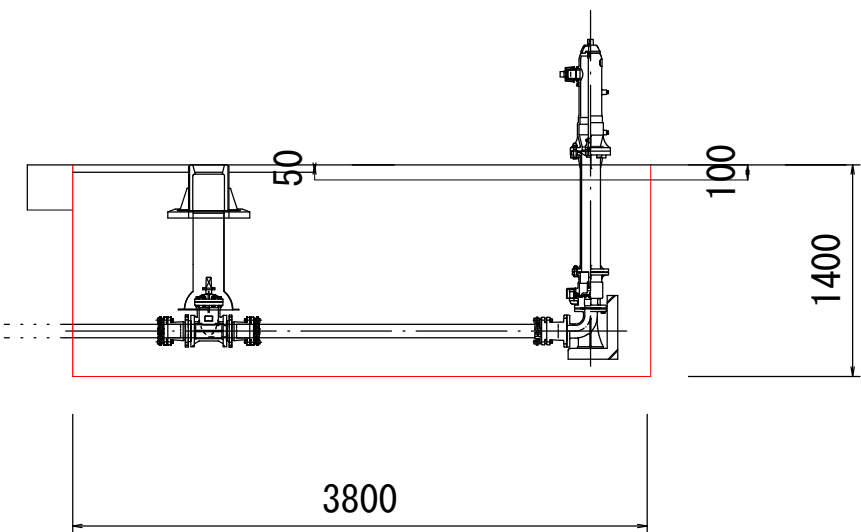
【掘削断面図】
