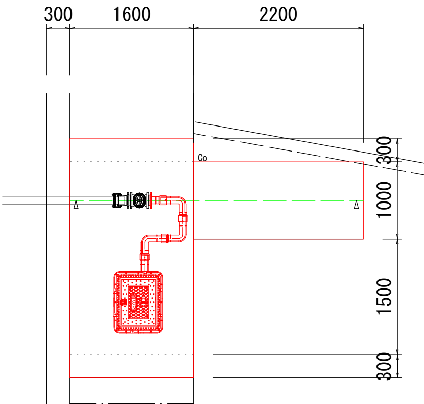
【復旧平面図】
