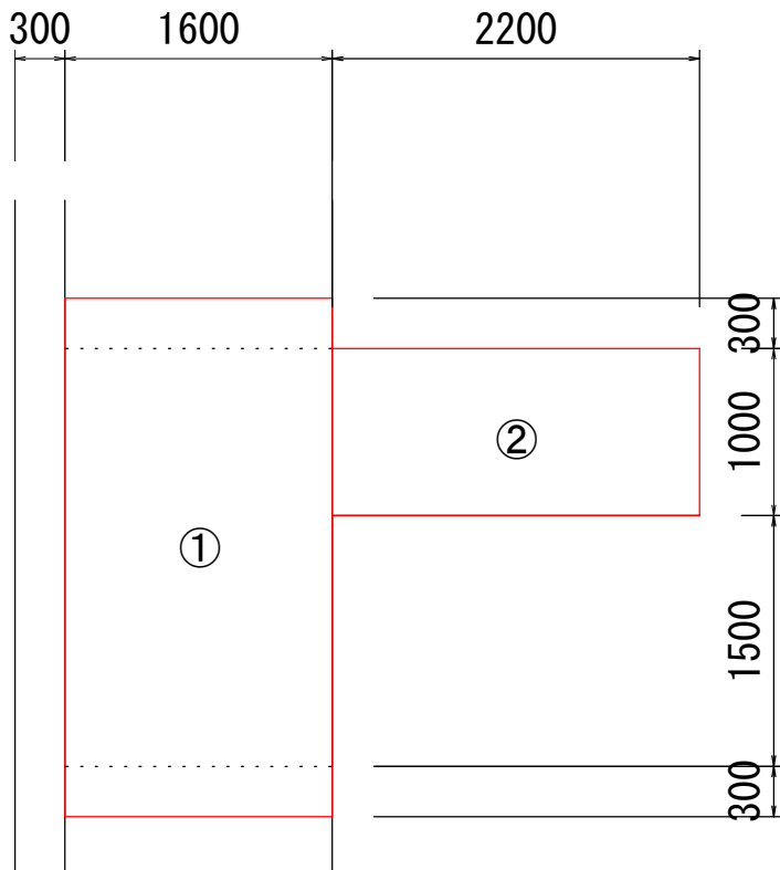
【掘削範囲分割】 S=1/50
