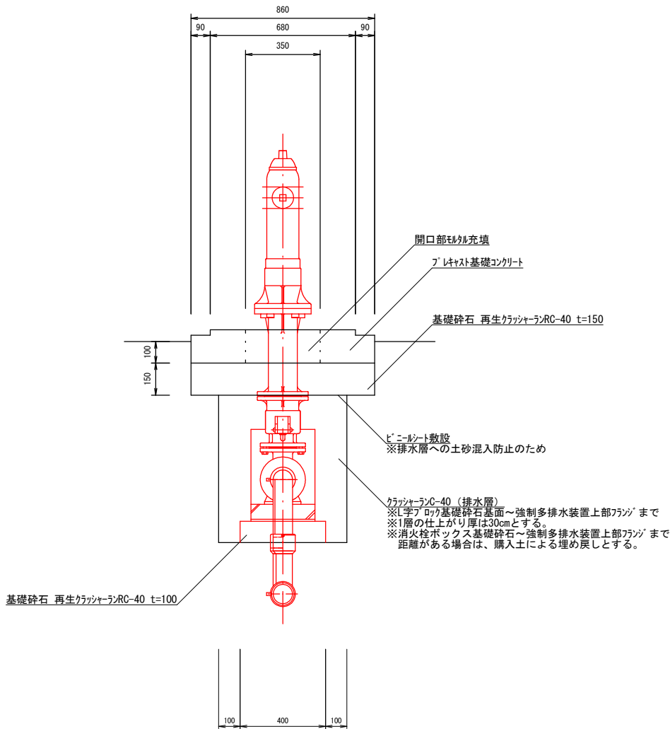
【正面断面図】
