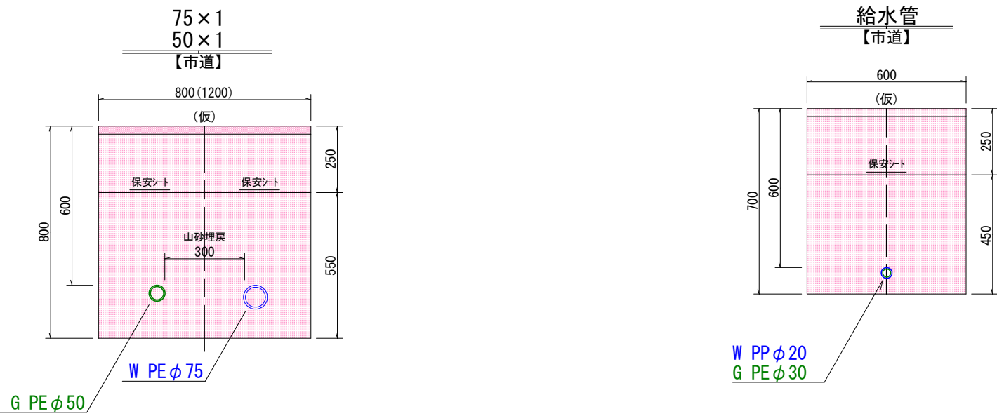
掘削標準断面図 S=1:20
