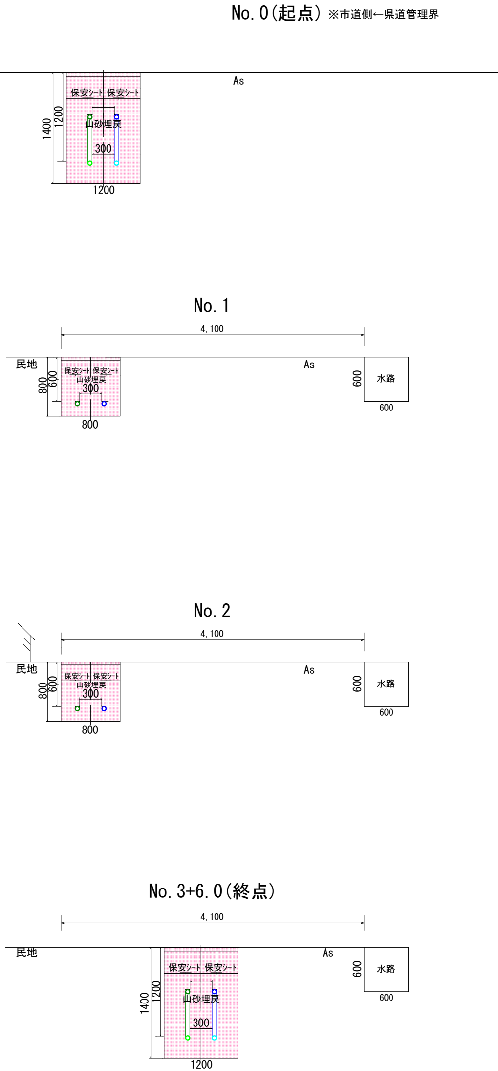
横断面図 S=1:50
