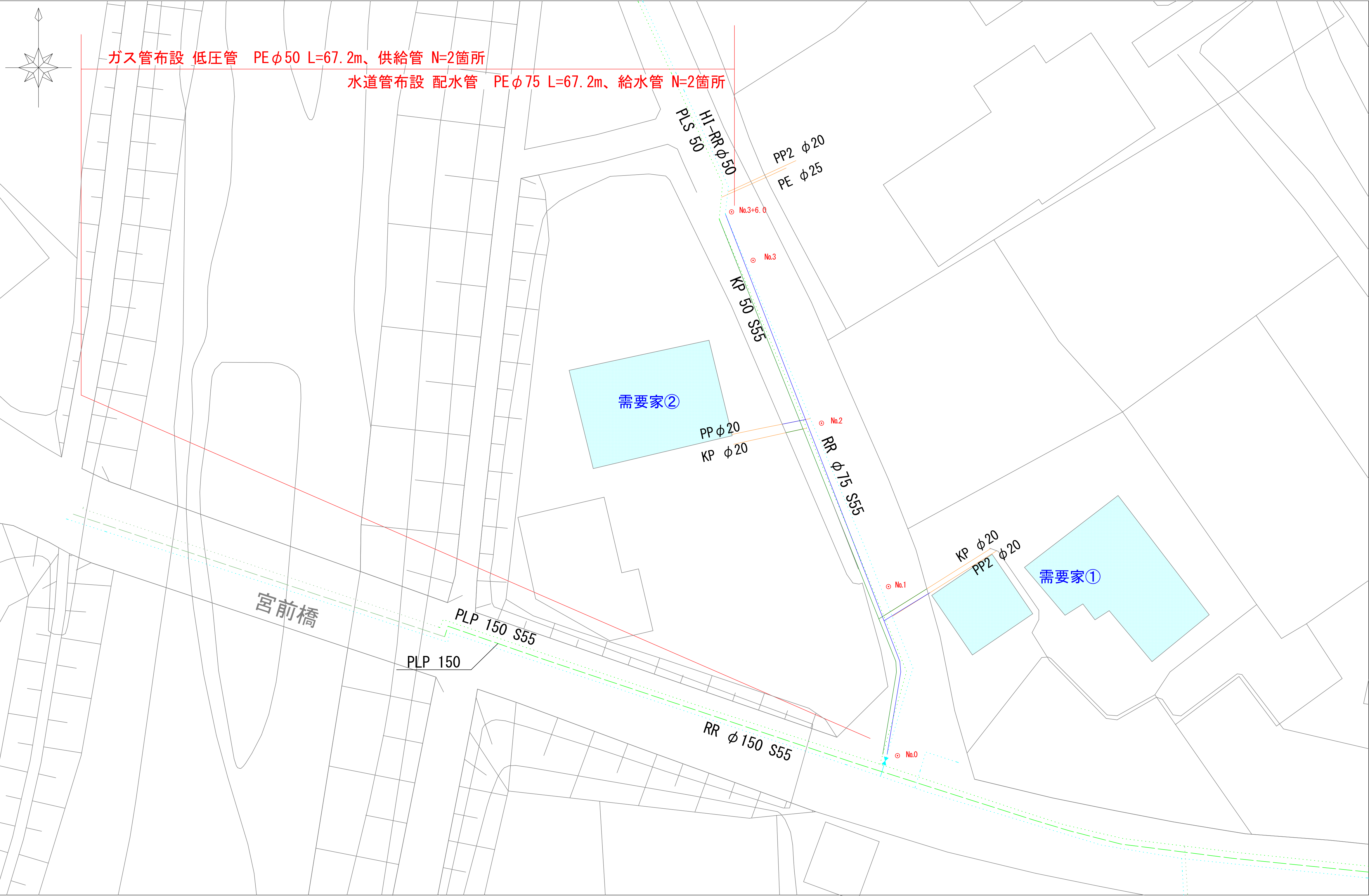
平面図 S=1:250
