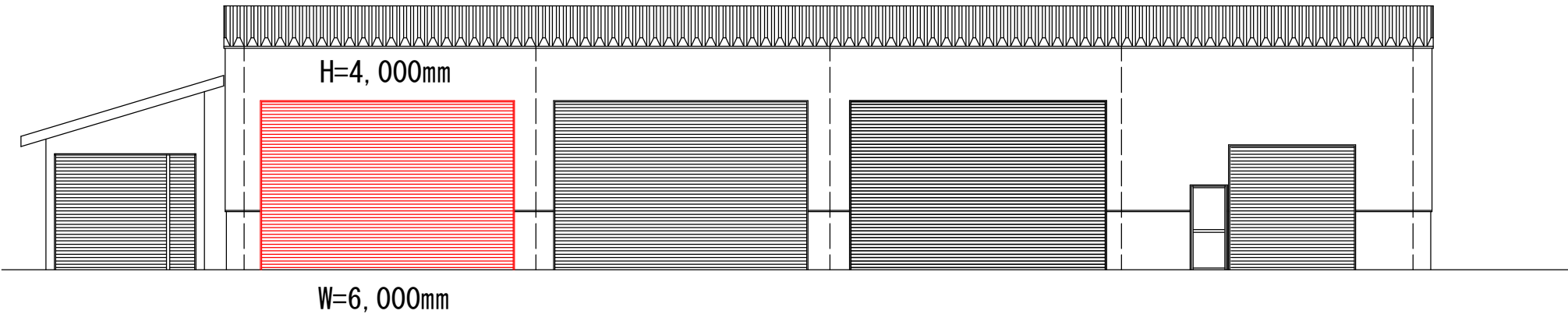
東側立面図 S=1/100
