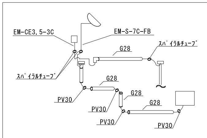
【配管図】
