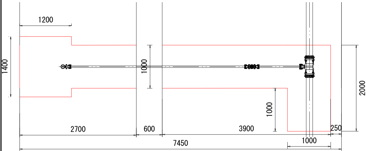
【掘削平面図】 S=1/50
