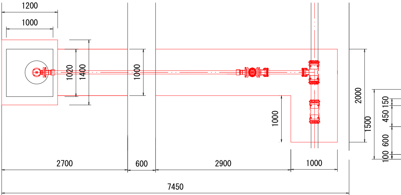
【復旧平面図】 S=1/50
