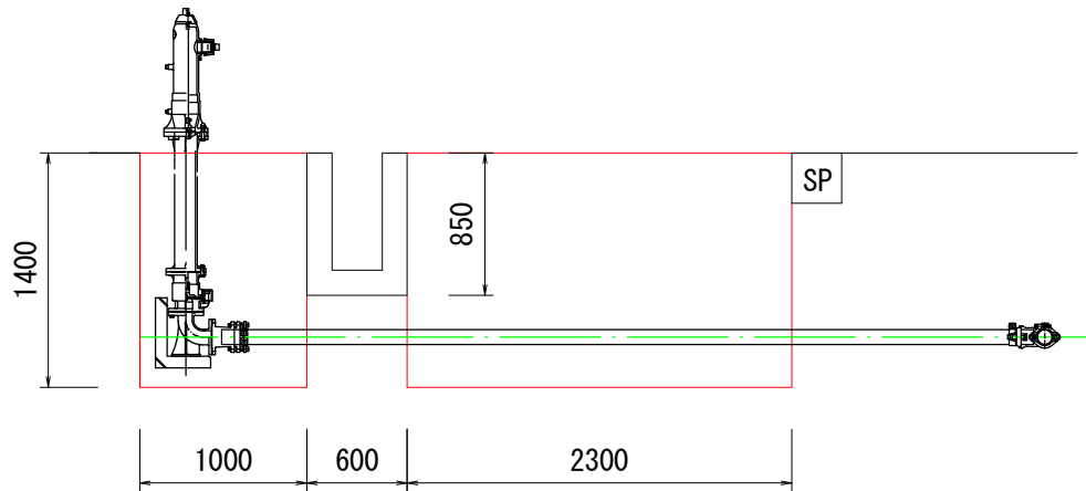
【掘削断面図】
