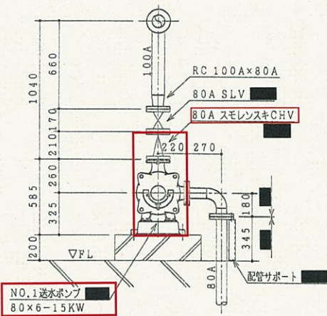
NO.1 ポンプ据付断面図
