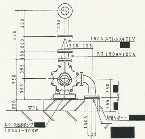
NO.2ポンプ据付断面図
