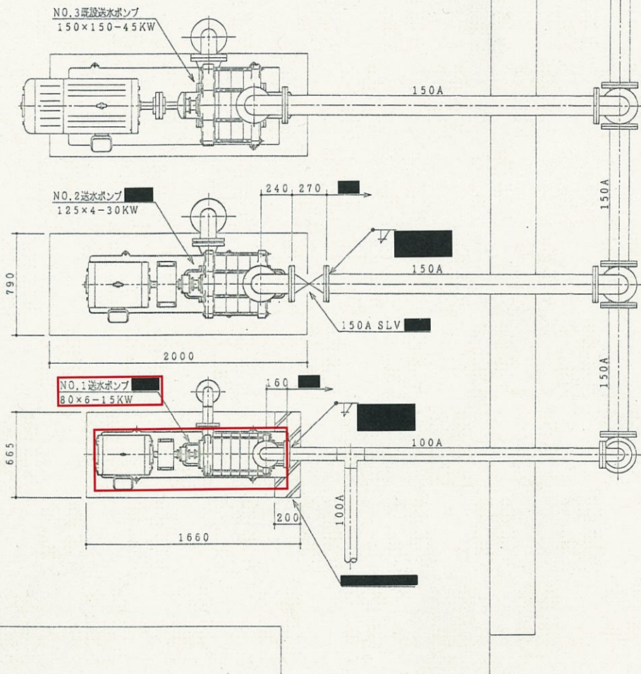
ポンプ据付平面図
