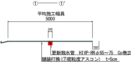
標準横断面図 S=Free
