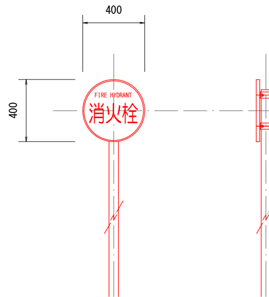
【水利標識寸法図】
