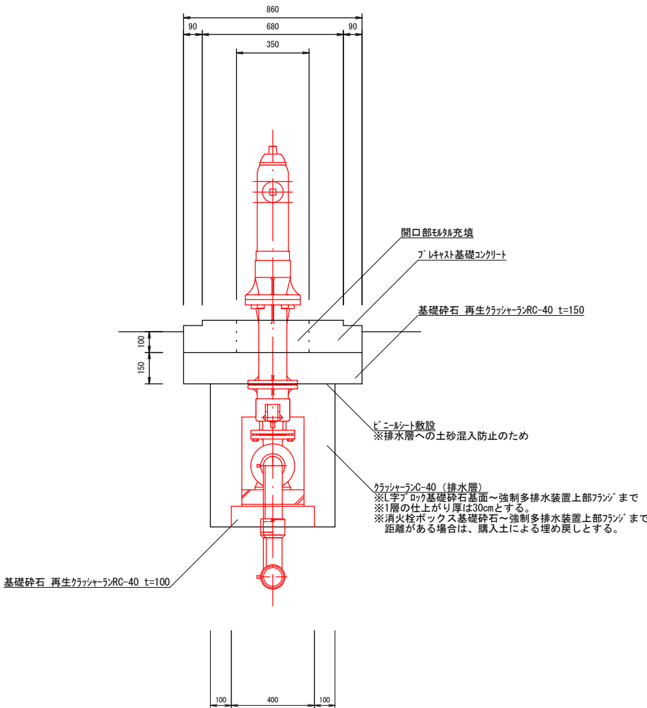
【正面断面図】
