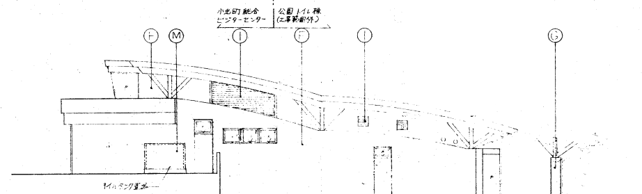
南側立面図
