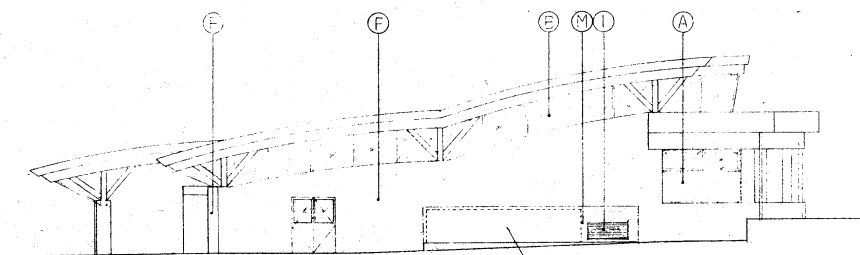
西側立面図
