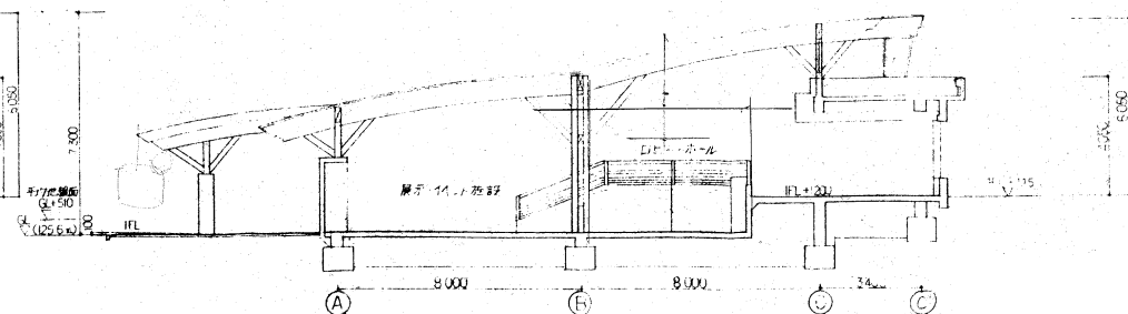
A-A断面図
