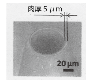
中空微小針の先端
