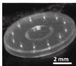
無痛注射針（中空微小針アレイ）の試作品。
