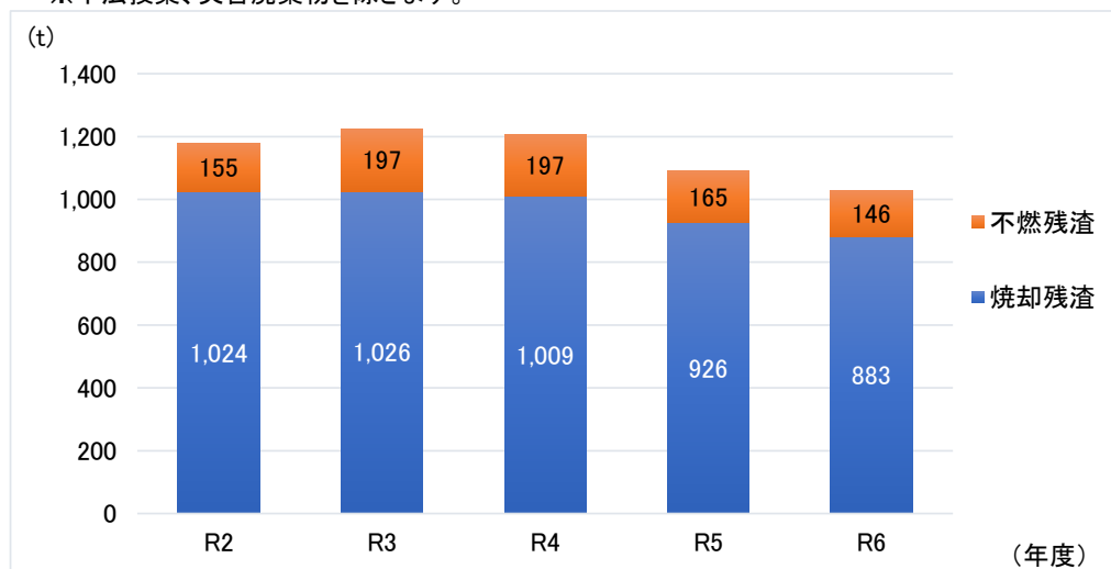
図 3-1-10 最終処分量の推移
