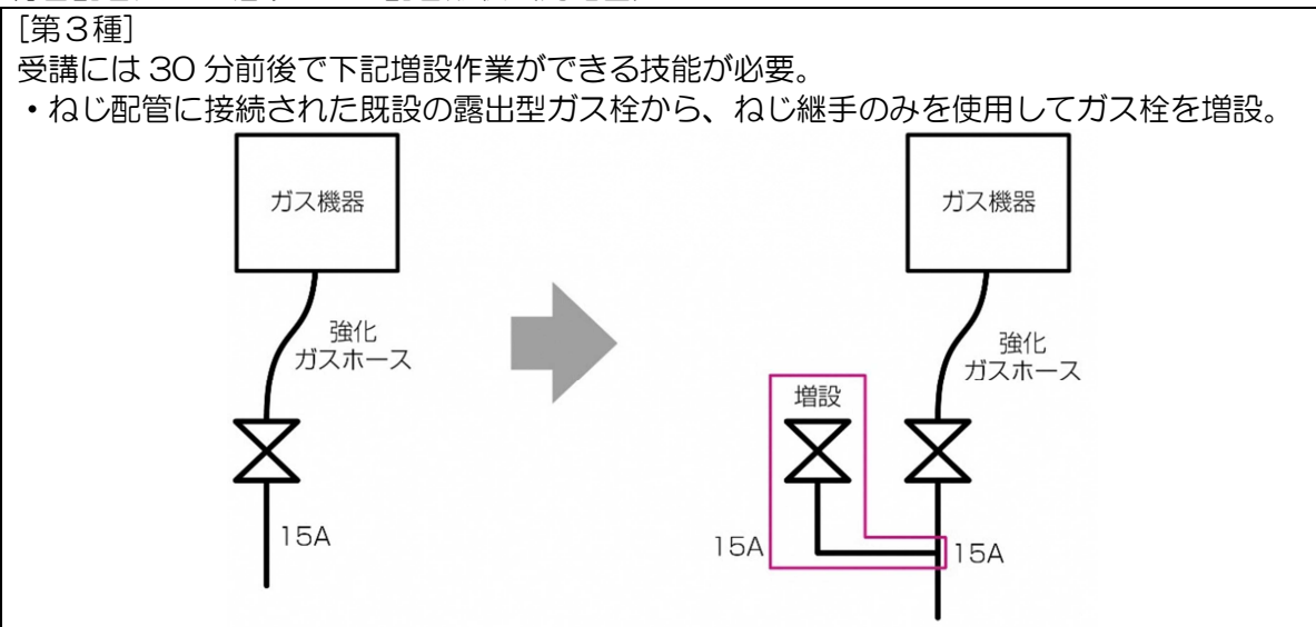
総合配管実習で組み上げる配管形状(簡略図) つづき
