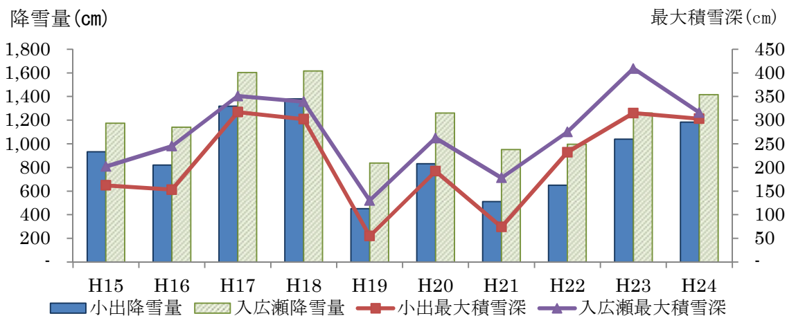
図3 年別降雪量 最大積雪深
