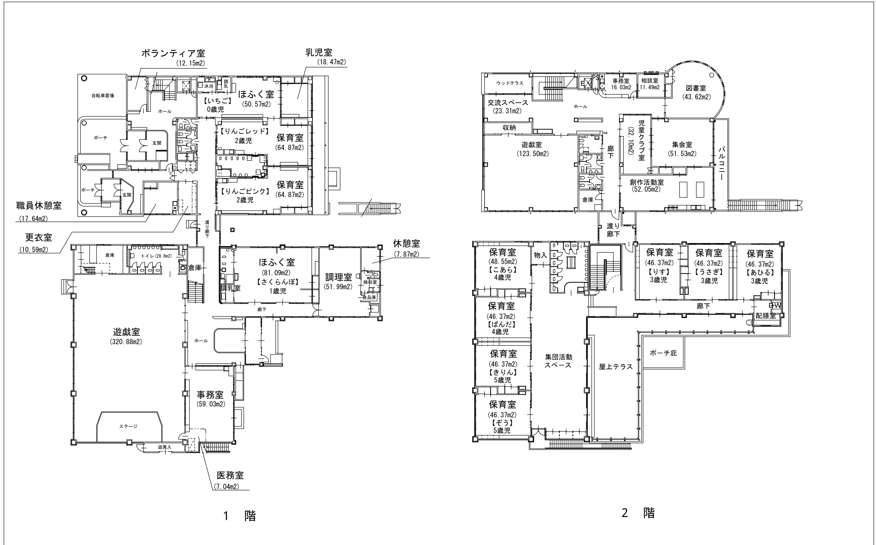
魚沼市立つくし保育園 平面図
